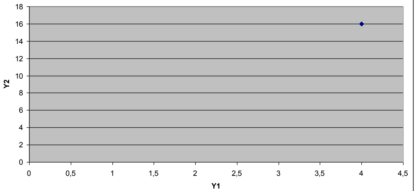
Gen 13 Ranking
