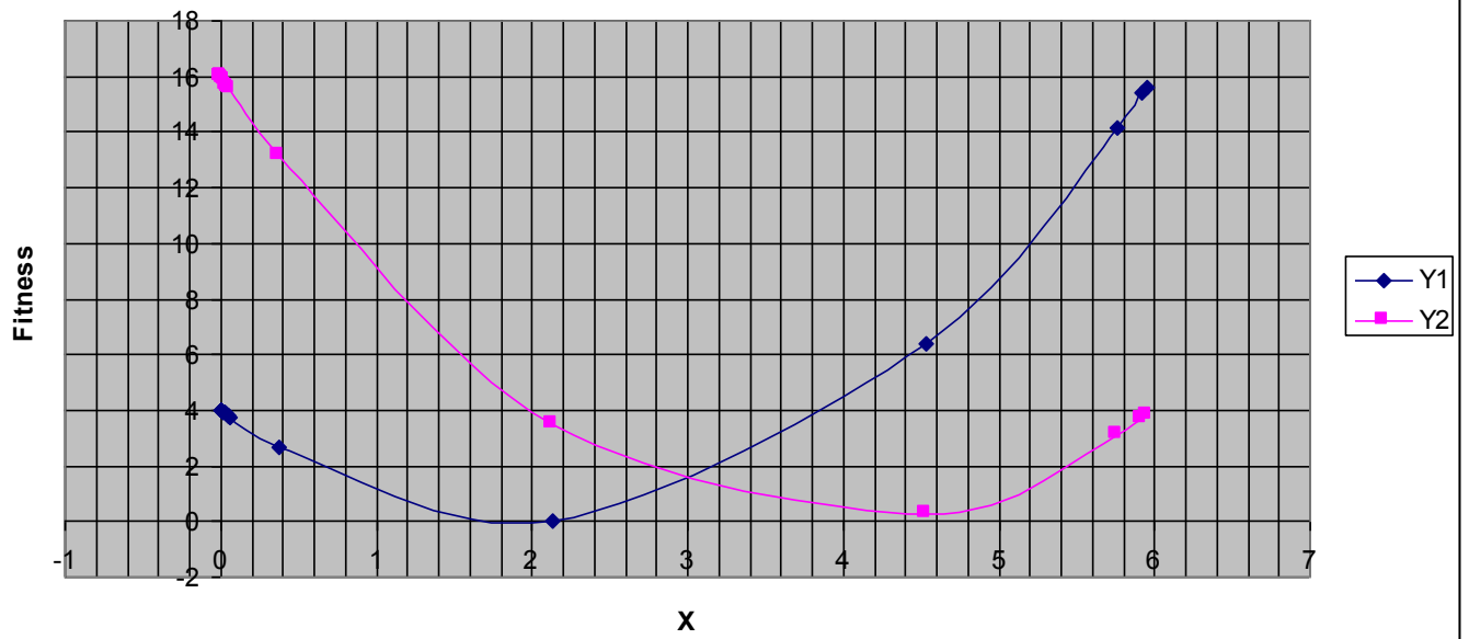
Gen 5 Ranking
