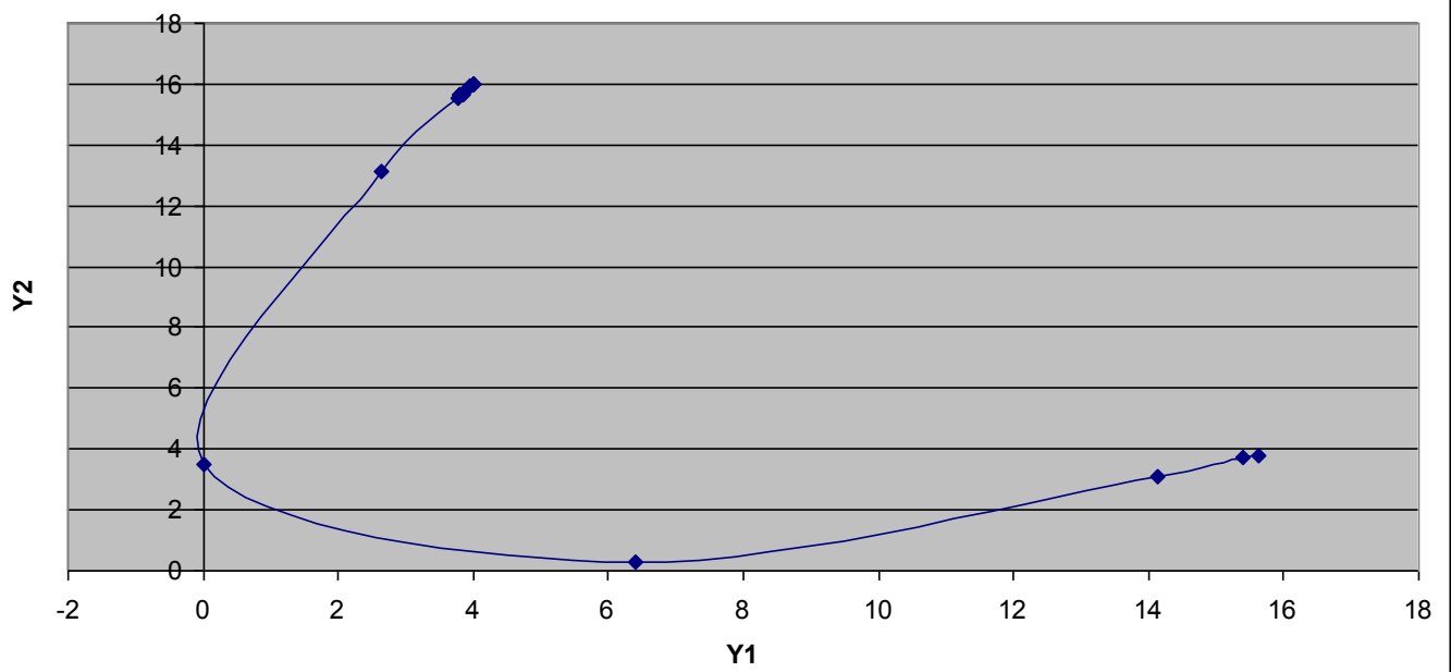
Gen 5 Ranking
