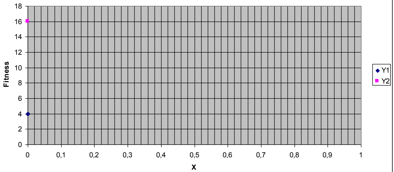
Gen 13 Ranking
